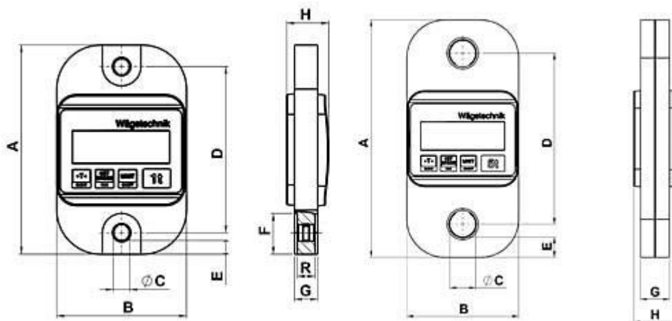
Afmetingen van de weeghaak TZR 1,0 t
