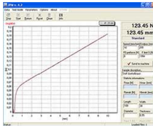
Software voor de universele controlemachine ZPM
