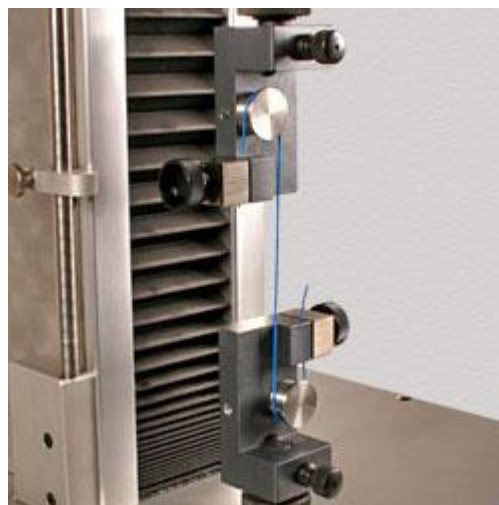
Universele controlemachine ZPM met kabelspanner
