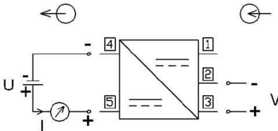
Aansluitschema van de signaalomvormer voor 0 - 10 V signaal PCE-P17U
