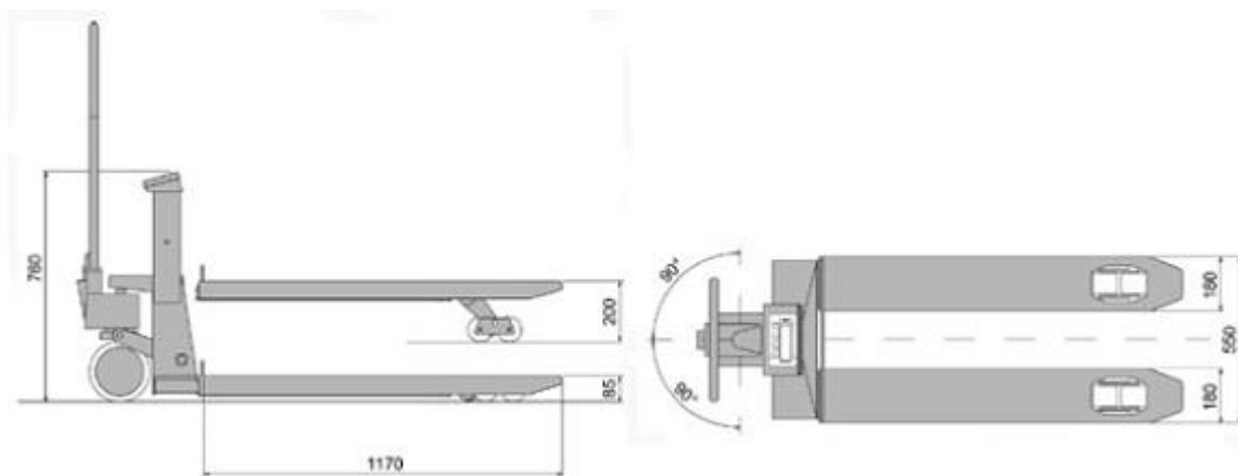
Afmeting van de palletwagen met weegschaal
