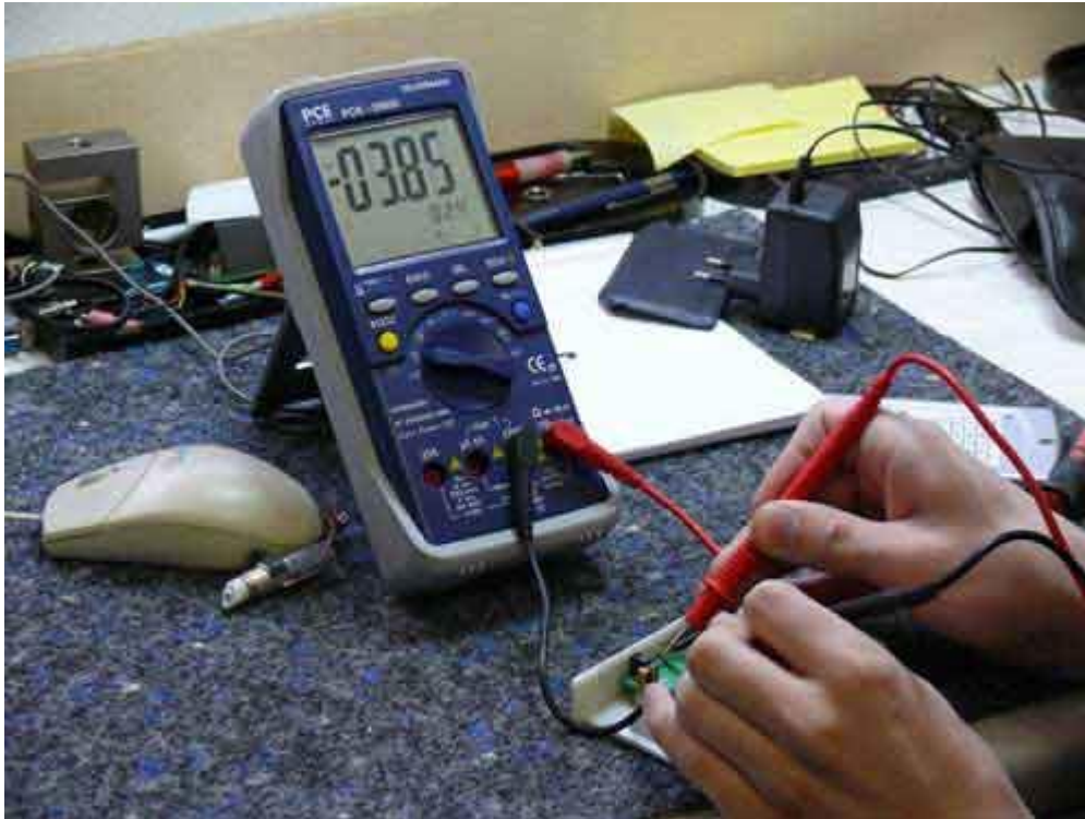
Hier ziet u de digitale multimeter PCE-DM 22 wordt gebruikt
