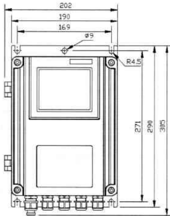
Afmetingen van het display van de Container weegschaal PCE-LWS Serie
